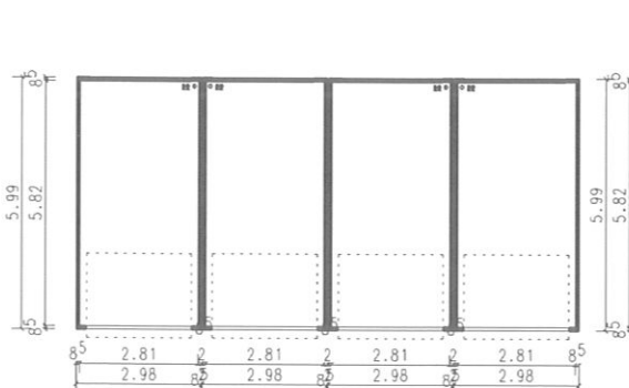
Reihengarage Typ 1, 2, 3
