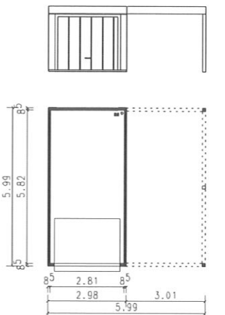
Garage und Carport Typ 1, 2, 3
