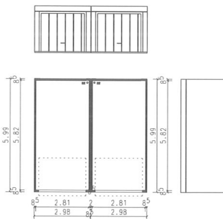
Doppelgarage Typ 1, 2, 3
