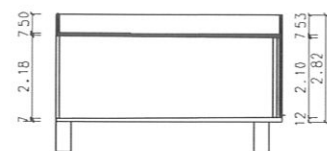
Garage mit Dachbegrünung Typ 1, 2, 3
