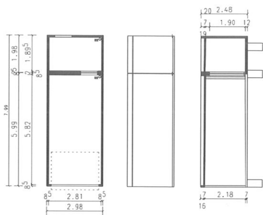
Einzelgarage mit Geräteanbau Typ 1, 2
