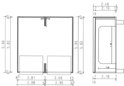
Raumgarage Typ 1, 2, 3
